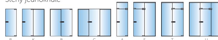
Stěny dvoukřídlé
